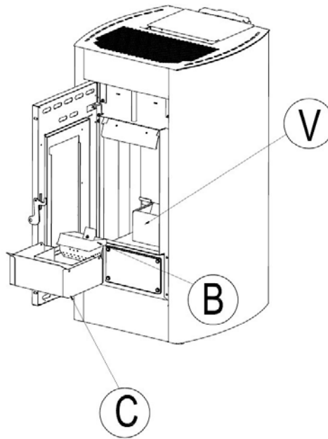
Fig. 33 - Reinigung
