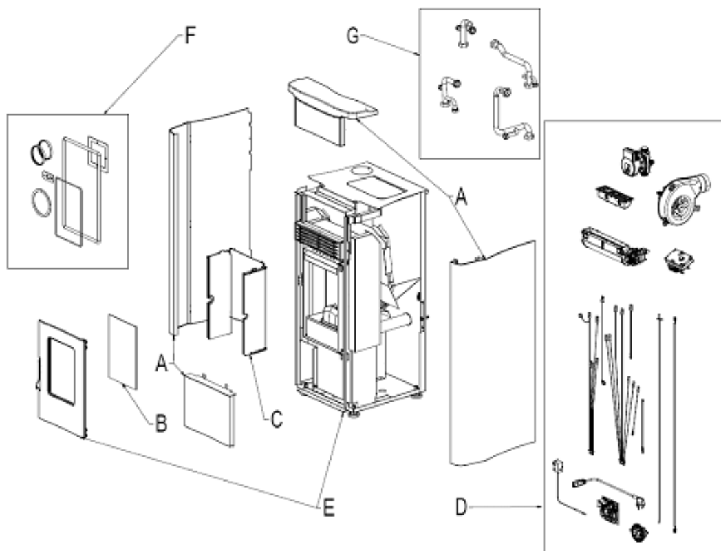
Fig. 1 - Explosionszeichnung
